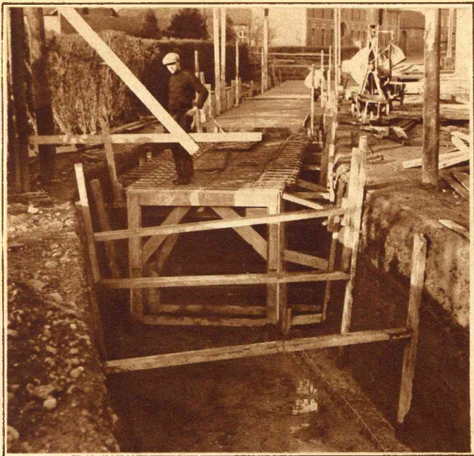
Met de overkapping van de Geleenbeek is men reeds gevorderd tot in het dorp zelf. Wanneer dit werk gereed zal zijn is het dorp verlost van de ongemakken en den minder lekkeren reuk van de open beek. Een kijkje in de overkapping.
