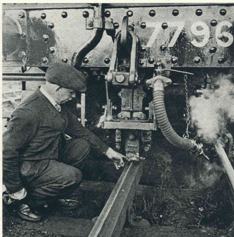
Door 'n Engelsche spoorweg-maatschappij worden momenteel proeven genomen met een instrument, dat het trein-verkeer bij zwaren mist sneller en reiliger zal maken. Over 'n elektrische rail, die met de seinhuisjes in verbinding staat, glijdt een aan de locomotief berestigde z.g. „schoen“, welke aan den machinist bij reilig verkeer een eentonig geluid en bij gevaar 'n dringend sirene-signaal doorgeeft. Bovendien kunnen uit de seinhuisjes in geval van nood de remmen van den trein automatisch in werking worden gesteld.
