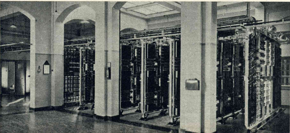
Het laatste snuffje op het gebied van de moderne telefoontechniek: de nieuwe automatisch werkende centrales, zooals men die in allerlei vorm en omvang in tal van plaatsen van ons land kan bewonderen en gebruiken.
