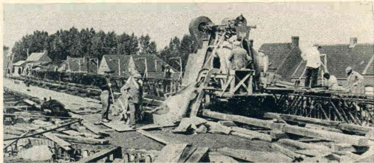
Het nieuwe viaduct te Roermond, dat een groote verbetering inhoudt in het moderne snelverkeer op den hoofdverkeersweg Roermond-Venlo-Nijmegen, nadert zijn voltooiing. De betondekking over de spoorlijnenoverbrugging wordt gestort. Een overzicht bij de werkzaamheden, die het verkeer in prettiger banen leiden, daar de overweg aan deze zijde vaker dicht dan open staat.
