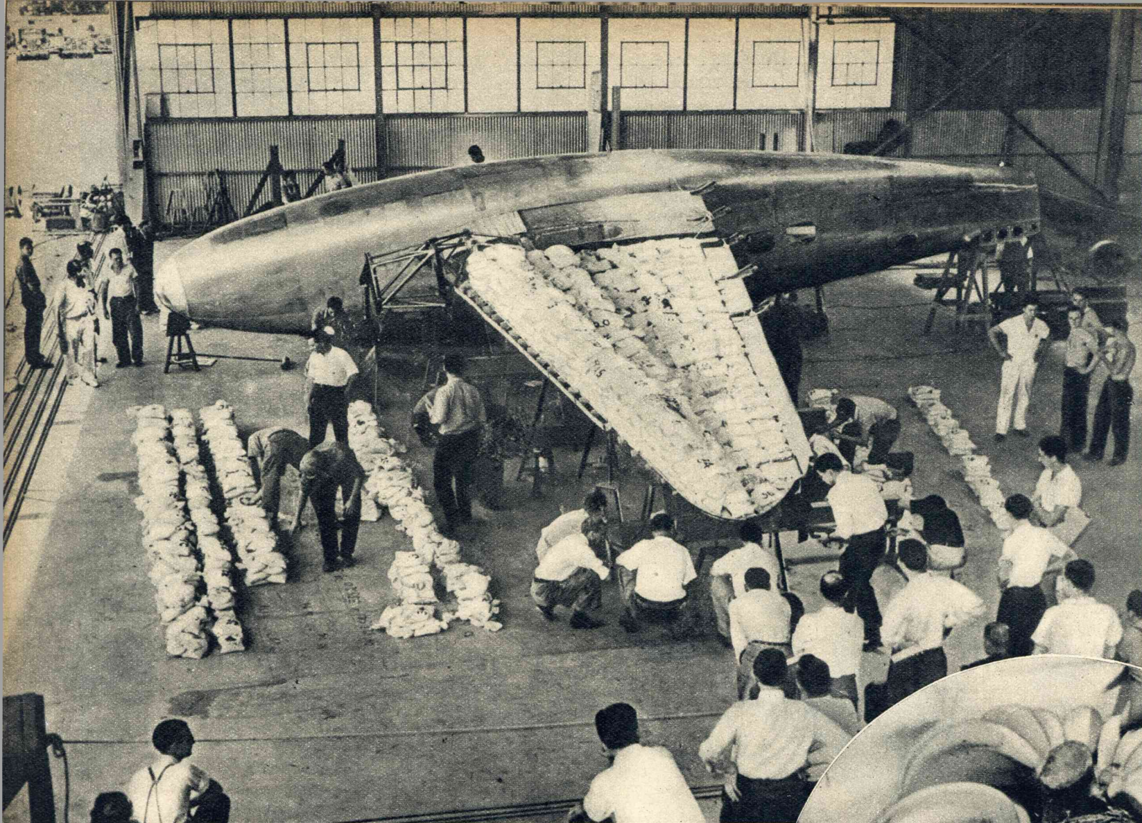
Een interessante foto in 'n vliegtuigenfabriek te Burbank (Californië). Alvorens het toestel wordt afgeleverd, belast men de vleugels met zakken zand tot een gewicht van 35.000 pond. Deze proefneming geschiedt in tegenwoordigheid van Amerikaansche regeeringsambtenaren, die het bewijs van luchtwaardigheid moeten afgeven.
