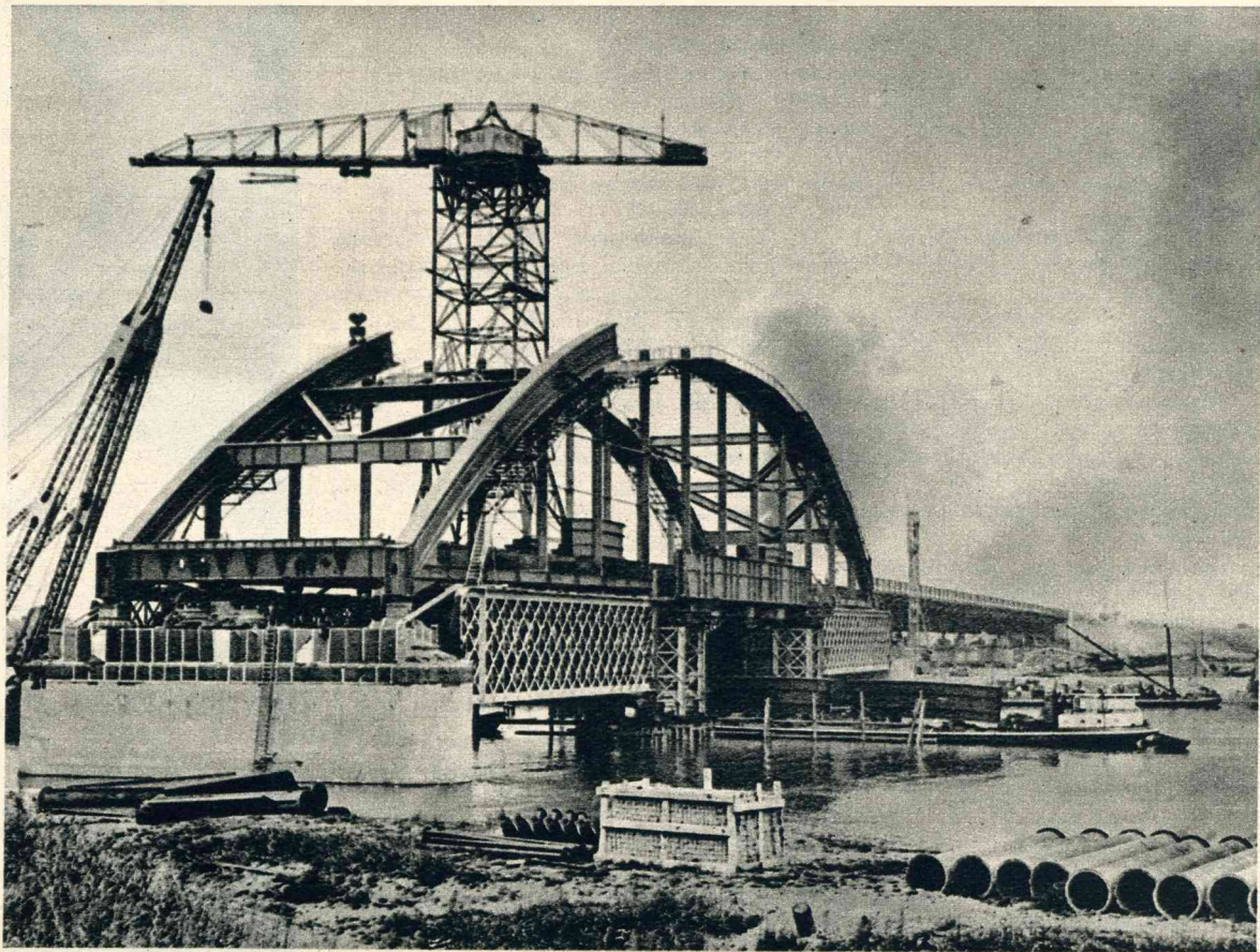
De nieuwe brug bij Hedel nadert haar voltooiing. — De groote, sierlijke boog, die de doorvaart overspant is bijna gereed, zooals we zien. Het geheel levert nu al een prachtig gezicht op.
