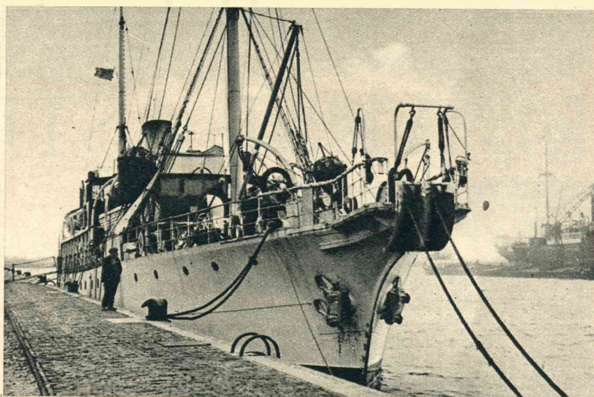
Een storing in den telefoonkabel tusschen Nederland—Engeland. Het Engelsche kabelschip Alert, voor reparatie te Vlissingen gestationneerd.
