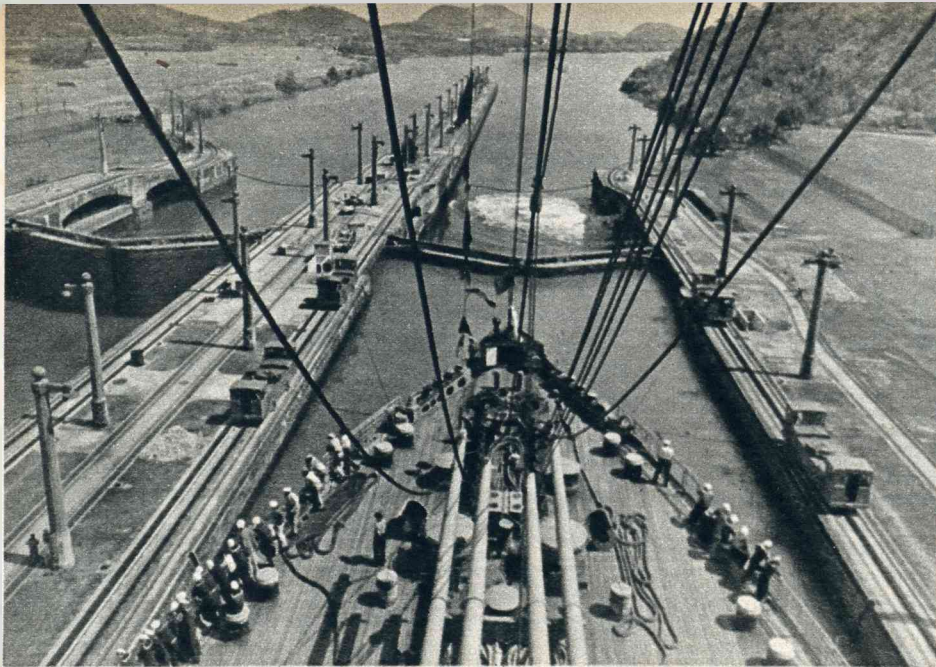
Tijdens het wachten in de sluizen. Op de damwanden ziet men de elektrische locomotieven, die de schepen door de sluizen trekken.
