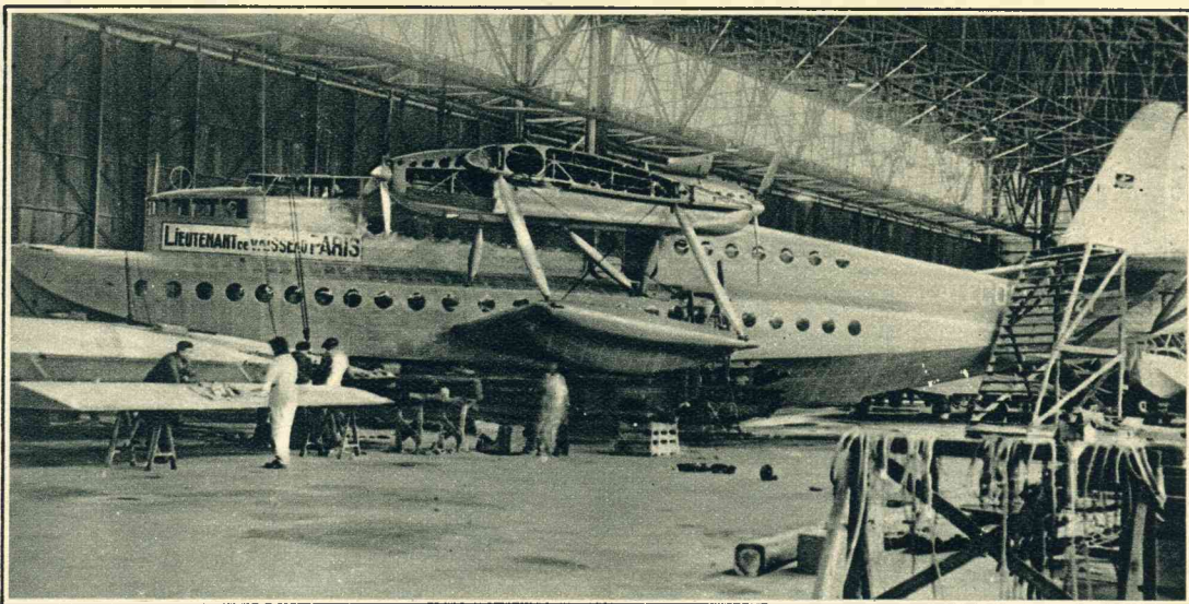
De „Luitenant de Vaisseau” in de werkplaatsen te Biscarosse (Zuid-Frankrijk), waar het schip gebouwd wordt. Bovenaan ziet men de „doorsnede” van den vleugel, waar deze verder aangebouwd wordt.
