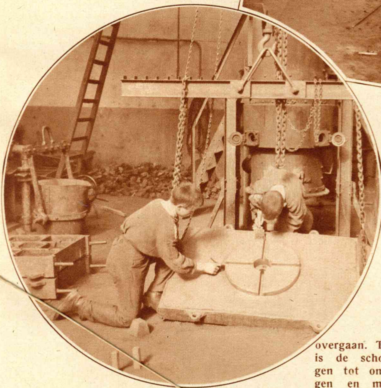
Het schoonmaken van een giestuk.
