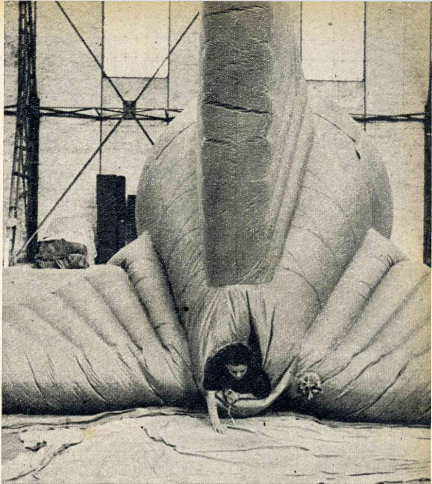
De ballonzijde wordt niet genaaid doch geplakt, wil de ballon volkomen luchtdicht zijn. De naden worden door speciaal daarvoor opgeleide arbeiders op dichtheid onderzocht nadat men den ballon niet met gas doch met lucht gedeeltelijk heeft gevuld.
