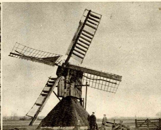
Twee standaardmolens in het Nederlandsche landschap, links het molentje achter de Kleverlaan te Haarlem, rechts een zogenaamd „spinkop”, een wipwatermolentje met binnenvijzel, in de buurt van Leeuwarden. Panorama-Valks
