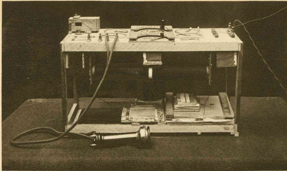
Ontvangstoestel met koppeling door inductie.
