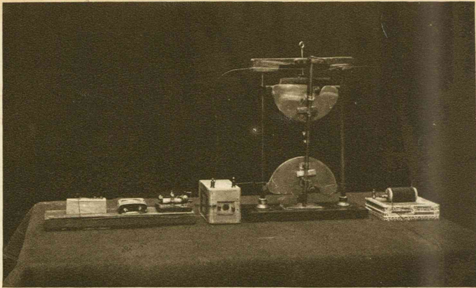
Een zender voor draadloze seinen (in beginsel).
