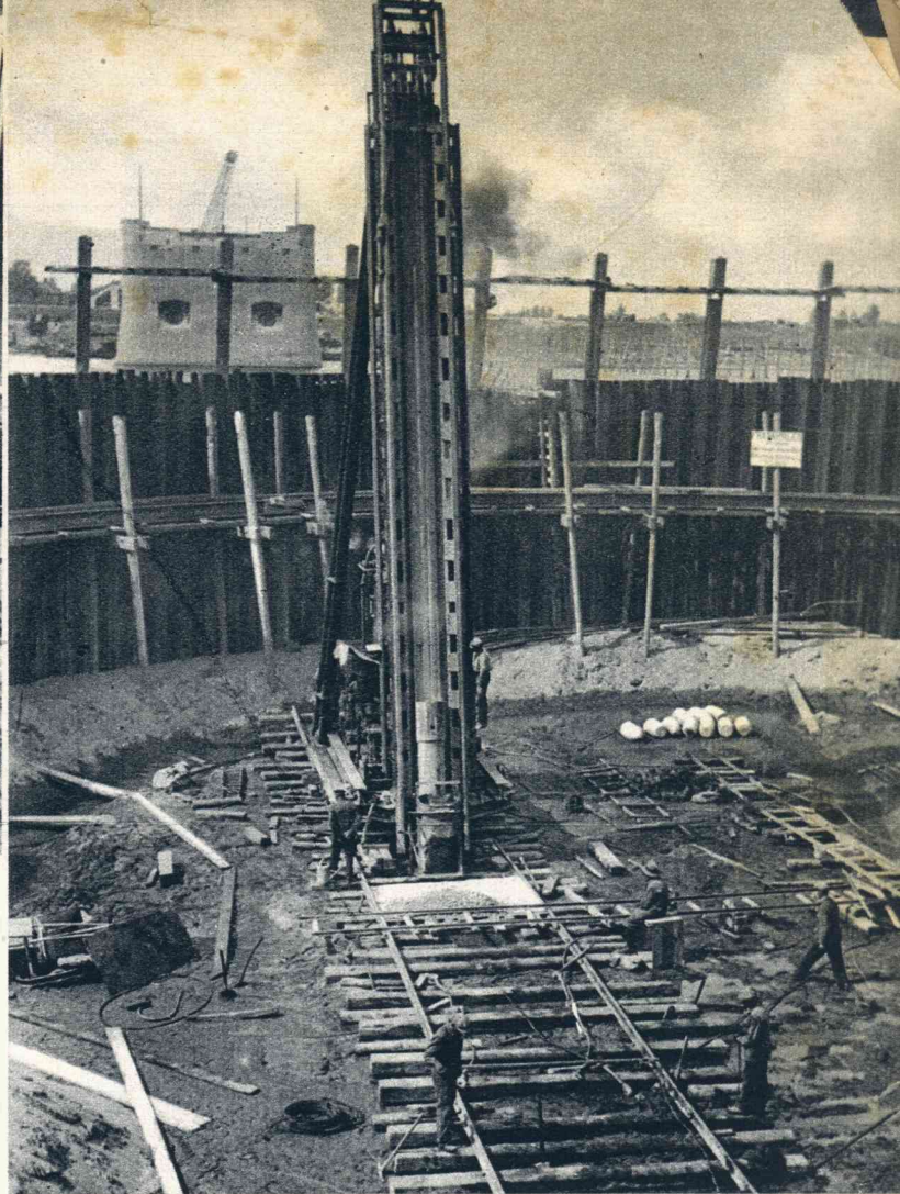
Een der bouwputten voor de Waalbrug bij Nijmegen is drooggemalen en 'n heistelling staat opgesteld voor het in den grond maken der betonpalen. Men onderscheidt de grootendeels ingeheidde stalen buis. Tegen den damwand een op jukken liggende stempelring.
