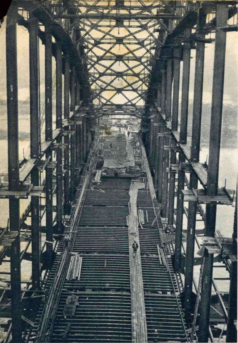
Aan den boog wordt de vloer opgehangen door middel van verticale hangstaven.
