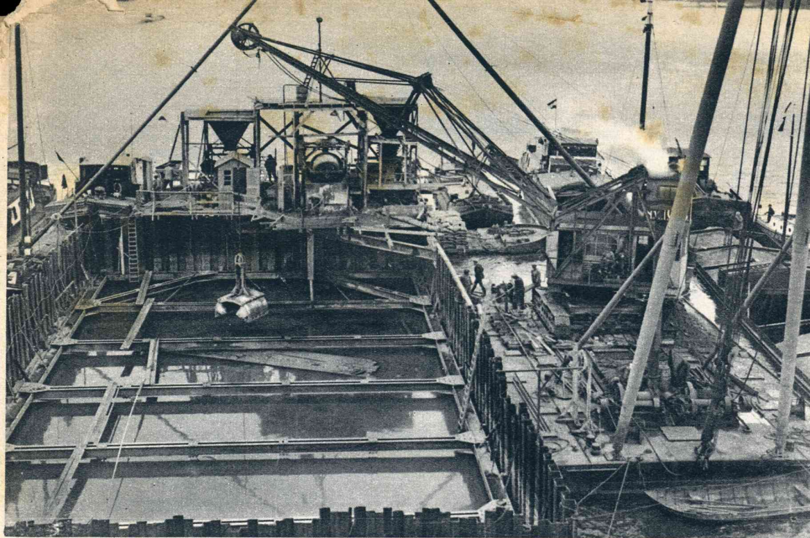
Door inheien van stalen damwandplanken is een bouwput gevormd, waarin juist onder water een betonplaat wordt gestort, waarna de put zal worden drooggepompt en de pijler opgebouwd. Om bij dit droogpompen te voorkomen, dat de wand door het buitenstaande water naar binnen wordt gedrukt, is een z.g. stempelraam aangebracht. Brug bij Zaltbommel.
