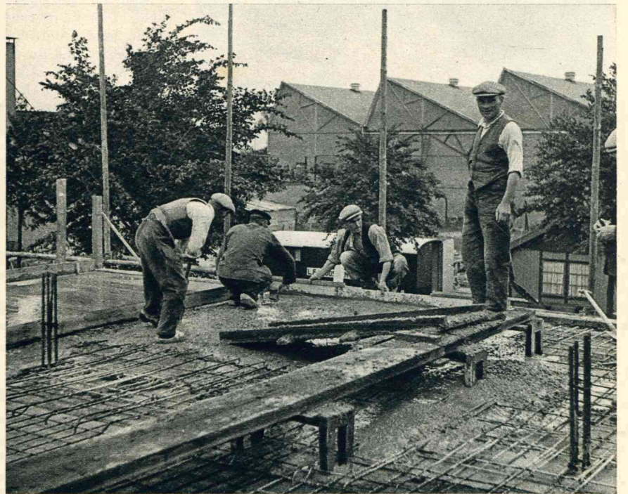
Door zware kolommen en balken gestut wordt een geheel betonnen verdiepingsvloer op de Vlissingsche brandweerkazerne aangebracht: wat er in Vlissingen ook afbranden mag, zeker niet het brandweerhuis.
