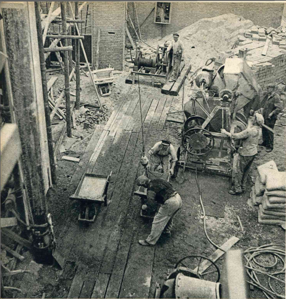
De Vlissingsche brandweer krijgt een modelhuisvesting: de nieuwe brandweerkazerne, die in aanbouw is, zal aan de hoogste eischen voldoen.
