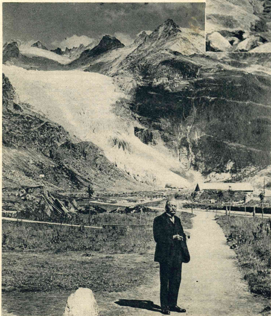
Het punt van oorsprong van de Rhône. Ruischend en schuimend zoekt het smeltwater van den Rhône-gletscher zich een uitweg door de reusachtige natuurlijke poort aan den voet van de ijsmassa.
