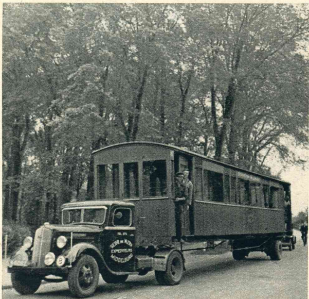
Een tweeslachtig voertuig — de tram op luchtbanden. Zoo werden de oude wagens van de Walchersche stoomtram, door maatschappij De Schelde aangekocht, bij gebrek aan rails naar Vlissingen vervoerd over den rijweg.
