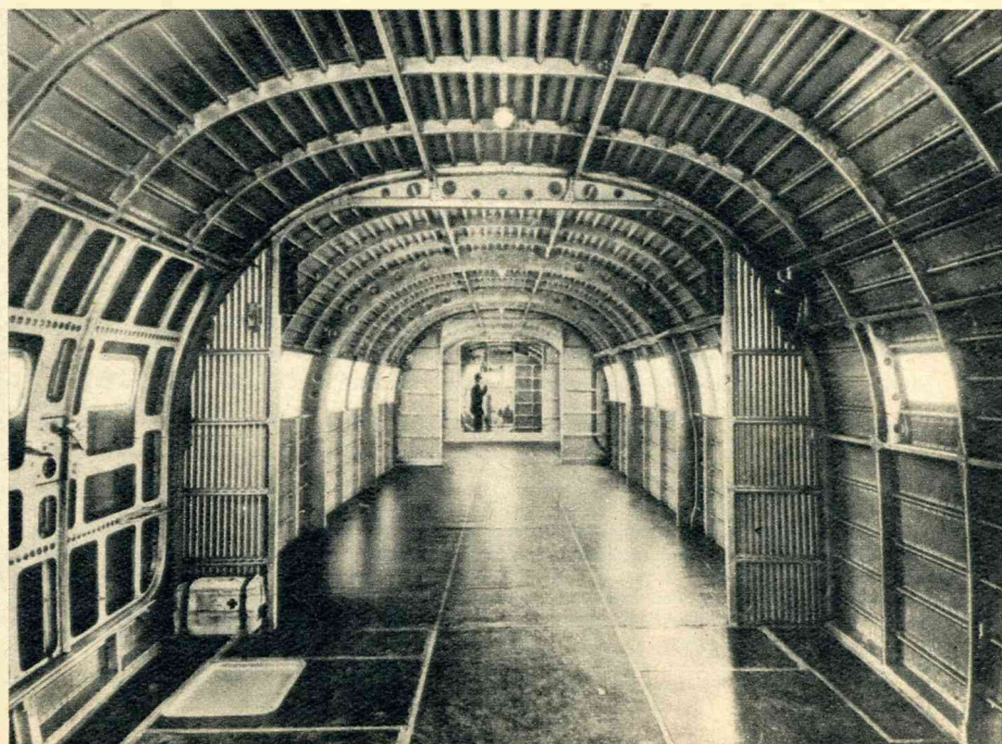
Het nieuwe viermotorige verkeersvliegtuig van de Junkerswerke te Dessau, dat dezer dagen is gereed gekomen. Het biedt plaats aan 40 passagiers, weegt omstreeks 22 ton en kan een snelheid bereiken van 400 km. per uur. Boven: de geweldige machine op het vliegveld. Onder: interieur van de enorme cabine.
