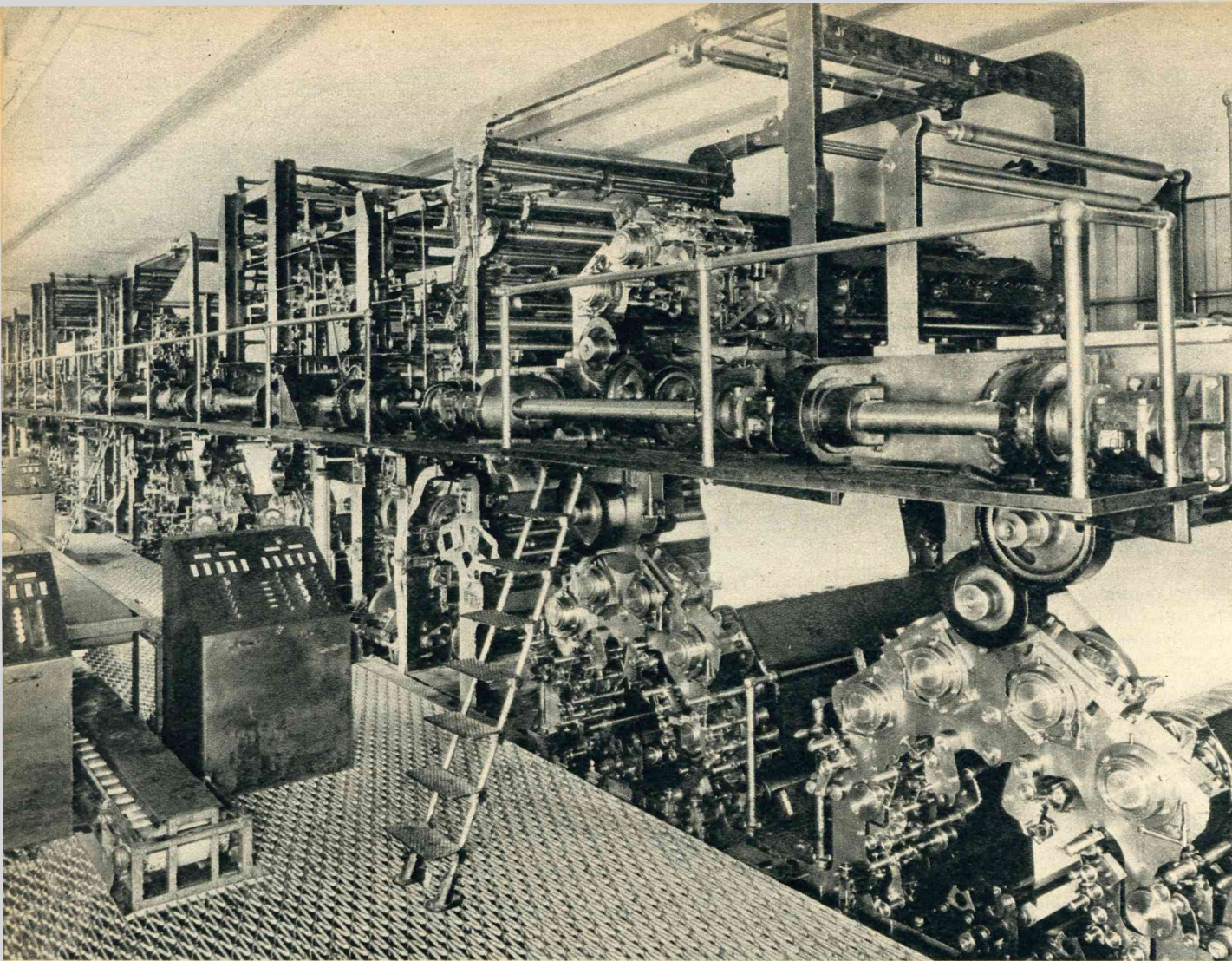
Een prachtig overzicht van de rotatiepersen van een grootbedrijf. Op deze machtige persen worden de mooie drie-kleurendrukken vervaardigd.
