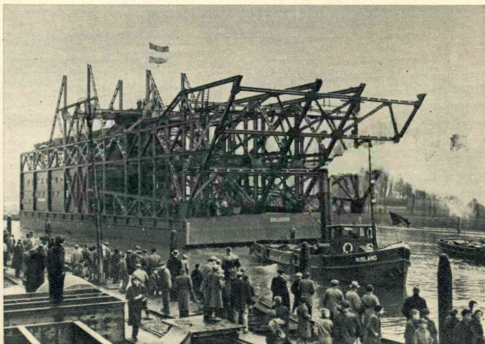
Zaterdag is te Kinderdijk de „Doejoeng” te water gelaten. Het is te hopen dat deze „grootste tinbaggermolen ter wereld” ’n voorspoediger reis heeft naar de Indische wateren dan zijn voorganger „Kantoeng”, die, zooals men zich herinneren zal, nauwelijks onderweg zijnde vergaan is.
