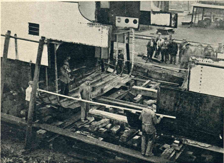
Op de werf der Arnhemsche Stoomsleephelling te Arnhem wordt het instructie-vaartuig Prinses Juliana vergroot. Het schip werd daartoe doormidden gesneden, waarna de helften van elkaar werden getrokken.
