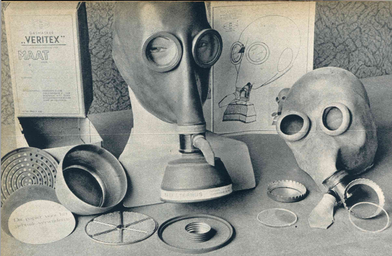
Een compleet masker, met de losse onderdeelen er omheen verspreid.
