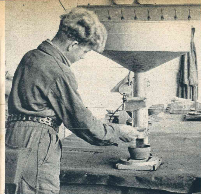
De groote ronde trechter is gevuld met actieve kool, waarvan een afgemeten hoeveelheid door het openen van een schuif in de filterbus terecht komt. Half verborgen achter den trechter de kwartslamp, die bij de controleering van de bussen een eventueel lek in het nevelfilter aan het daglicht brengt.
