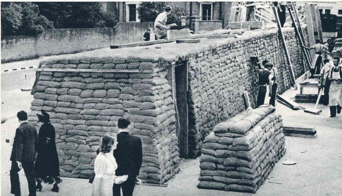
Een openbare schuilgelegenheid te Haverstock Hill: de zandzakken worden op hun plaats gehouden door kippengaas, ijzeren stangen en latwerk.
