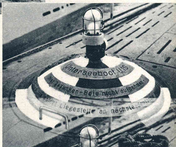
Een telefoonboei. Deze wordt, als de duikboot is gezonken, van binnen uit losgemaakt en drijft dan naar de oppervlakte. Door een telefoon kan men dan met de opgesloten bemanning spreken.
