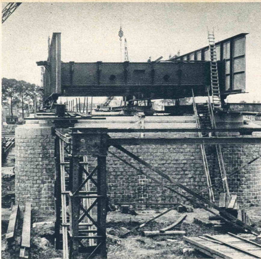
Het eerste gedeelte van de ijzerconstructie voor de vaste brug over den IJssel te Deventer werd geplaatst.
