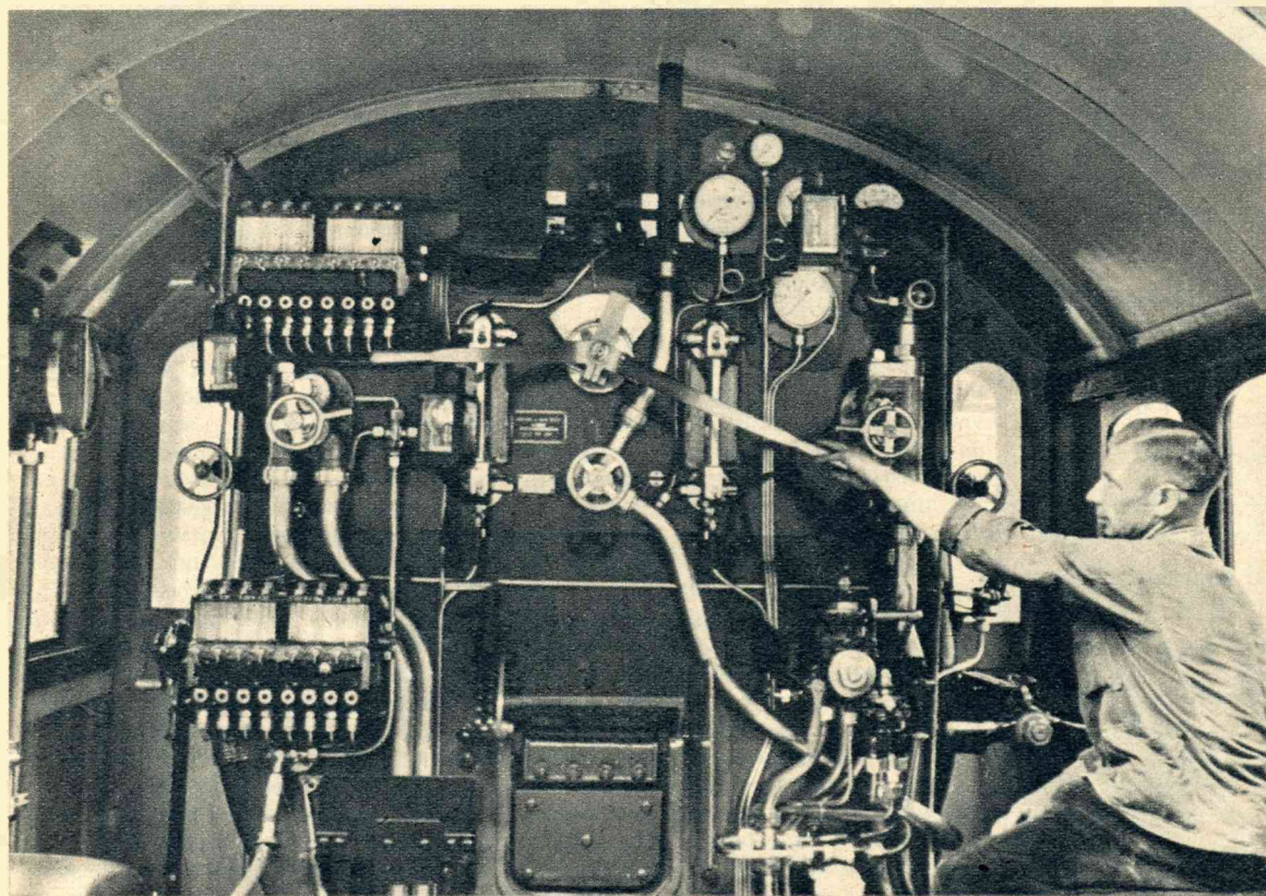
Hier ziet u de omvangrijke apparatuur in de cabine van een moderne stoomlocomotief, zooals er een in de tentoonstellingshal aanwezig is.
