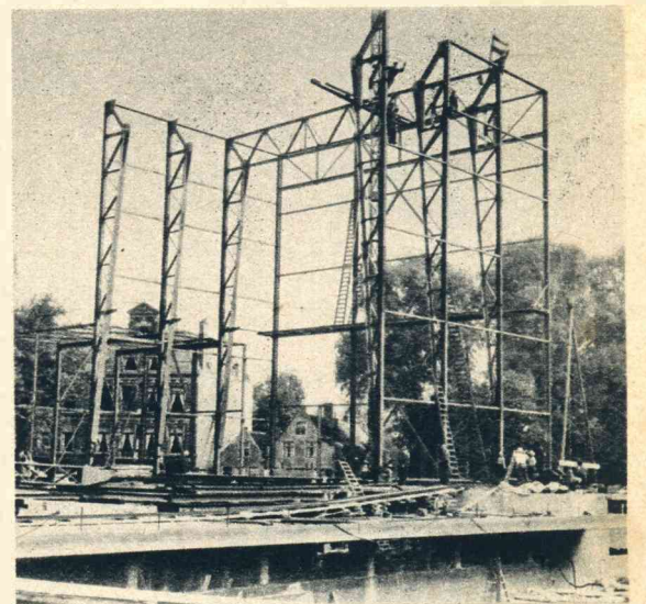
Het eerste spant voor Utrechts nieuwen schouwburg werd geplaatst en bij deze gelegenheid ging natuurlijk de vlag in top.
