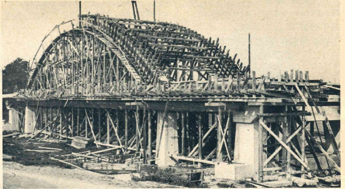
De oude Lingebrug te Geldermalsen zal spoedig verdwijnen. De bekisting voor de nieuwe oeververbinding is bijna gereed, zoodat men binnenkort kan aanvangen met het storten van beton.
