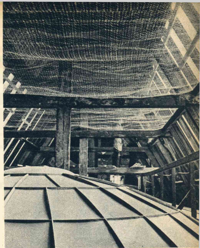
Over de hanebalken, die met een brandwerende verslaag zijn bedekt, is een vierdubbel net van ijzergaas gespannen om eventuele brandbommen op te vangen. Op deze manier hoopt het Groningsch museum van oudheden het ontstaan van brand te voorkomen.
