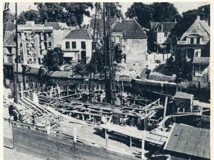
De bouw van een nieuwe brug bij de Diezerpoorten te Zwolle vordert gestadig en dit overzicht geeft een goed beeld van den huidige stand van zaken.
