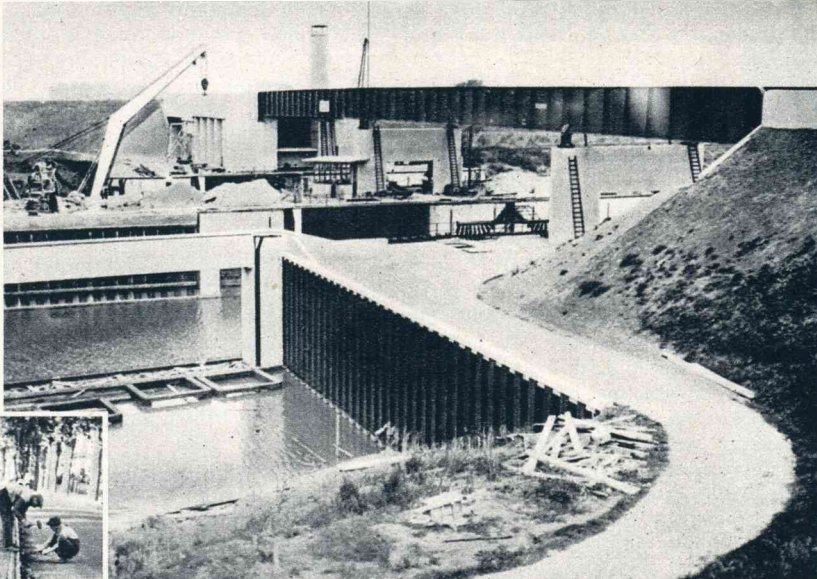
De dubbele schutsluis in het Amsterdam-Rijnkanaal te Ravenswaaij (Betuwe) is gereed gekomen. Voor het wegverkeer werd een brede brug over de sluis gelegd.
