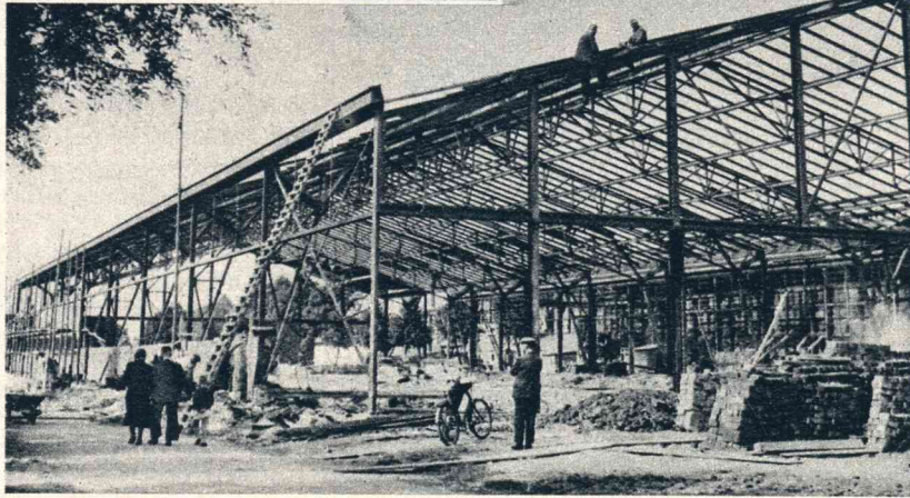
Op het Veemarktplein te Utrecht wordt een hal gebouwd, waarin tijdens het eeuwfeest der spoorwegen de directie het personeel zal ontvangen. Daarna wordt de loods gebruikt als garage van het Gemeentelijk Vuilnisbedrijf.
