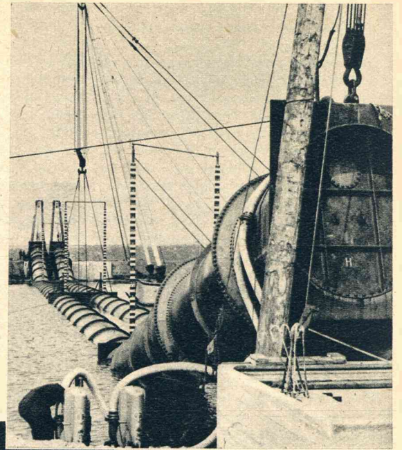
Groote duikers zijn neergelaten in het Amsterdam-Rijnkanaal onder IJphaa; door deze buizen zal het water van den Vaartschen Rijn gevoerd worden, die door het kanaal wordt gekruist.
