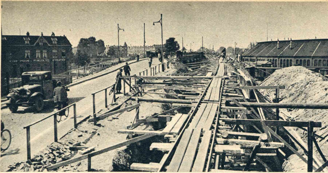
Er wordt met spoed gearbeid aan de verbreeding der Graafsche bruggen te Nijmegen, welke te smal waren en een lastige hindernis vormden voor het verkeer in de richting Den Bosch.
