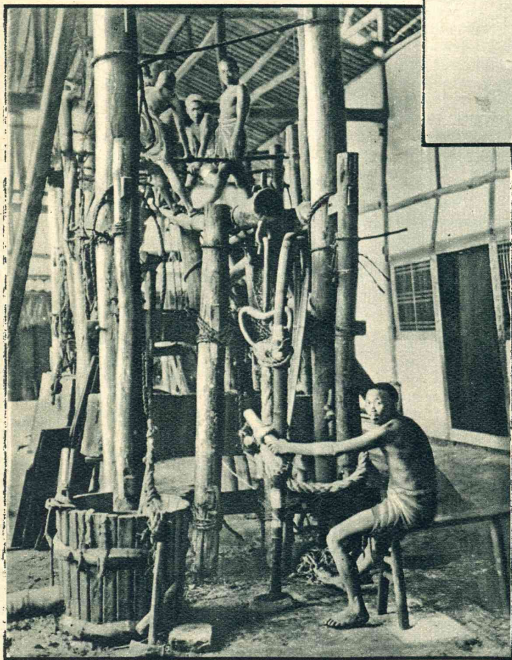
Waar de boor in den bodem verdwijnt; de inlander op den voorgrond draait den beitel af en toe een halven slag om; boven staan de arbeiders, die hefboom en boor beurte'ings opheffen en laten vallen.
