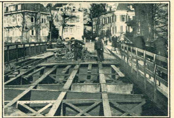
De Diaconessenbrug te Arnhem wordt gerepa-reerd en van een nieuw brugdek voorzien.
