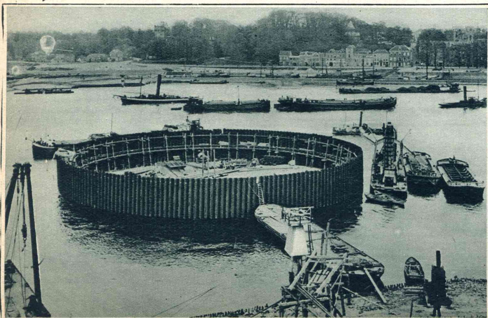
De overbrugging van de Waal bij Nijmegen. De bouwput aan den Lentschen kant is gereed; men kan nu beginnen met het bouwen van den eersten pijler in de rivier.
