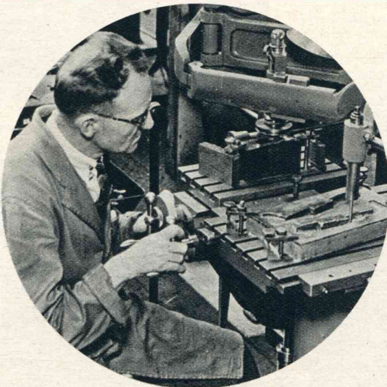
Dit is een voorbeeld, hoe de stalen stempels voor 't persen der metaalplaten in de gewenschte vormen worden gereedgemaakt. Met de grootste nauwkeurigheid tast de spil op den rooigrond het gesneden model van een vliegtuigromp af, en de machine fraist er op den achtergrond in staal een verkleining van.
