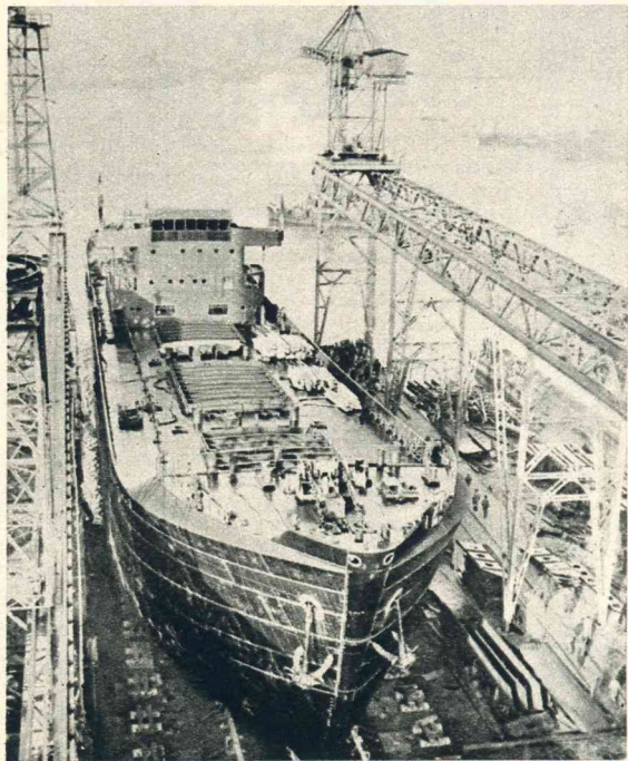
Van de scheepswerf P. Smit Jr. te Rotterdam werd met succes te water gelaten het motorvachtschip, bouwnummer 512. Het schip, dat later nog een naam zal krijgen, is bestemd voor de Steenkolen Handels- vereniging.
