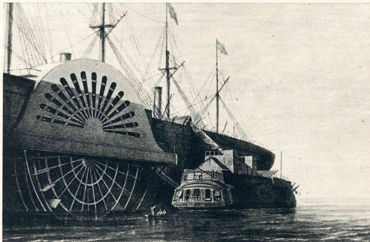
Een der geweldige schepraderen van de „Great Eastern”. Langs zij ligt een oud fregatschip, geladen met den transatlantischen kabel, die in 1866 door de „Great Eastern” tusschen Engeland en Amerika werd gelegd.
