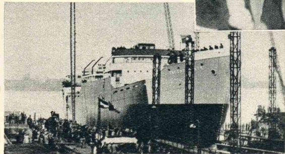
Onder groote belangstelling werd van de helling der N. V. Boele's Scheepswerven en Machinefabriek te Bolnes het dubbelschroefmotorschip „Inconfidente" met succes te water gelaten. Het schip werd gebouwd voor den Zuid-Amerikaanschen staat Rio Grande do Sul.
