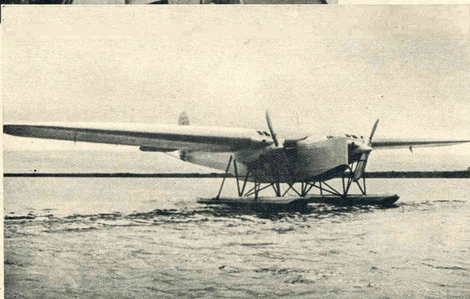
Het tweemotorige Fokkervliegtuig T I, dat in Indië verongelukte. De vijf inzittenden kwamen bij deze ramp jammerlijk om het leven.
