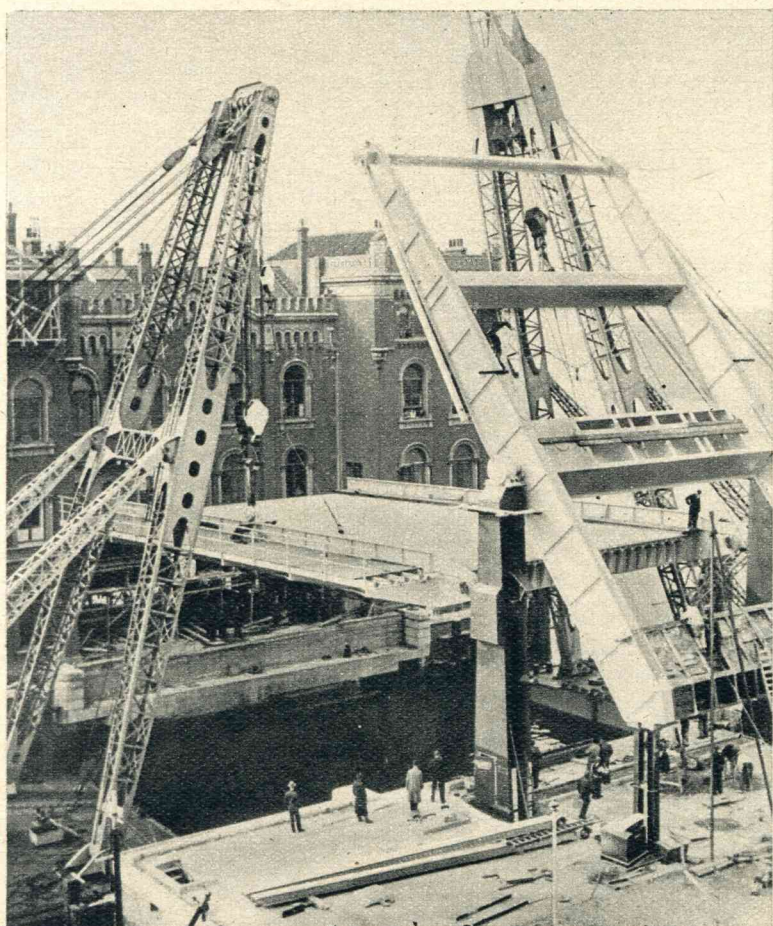
De grootste klapbrug van Europa werd Zaterdagmorgen over de Binnenhaven te Rotterdam geplaatst.
