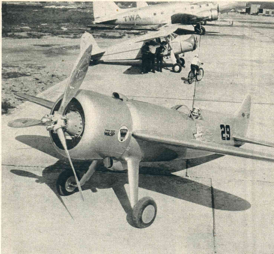
Bij de Benoix Trophy Race bereikte col. Roscoe Turner — bekend uit den wedstrijd Londen-Melbourne — met dit kleine vliegtuig een snelheid van 640 km. per uur.
