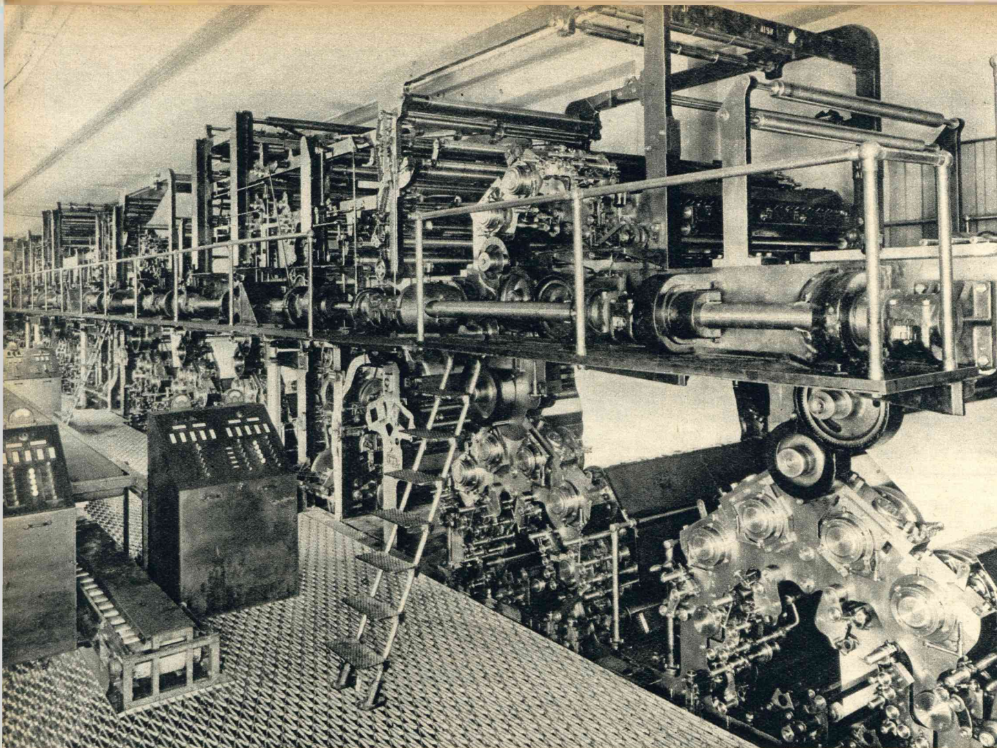
Een prachtig overzicht van de rotatiepersen van een grootbedrijf. Op deze machtige persen worden de mooie driekleurendrukken vervaardigd.
