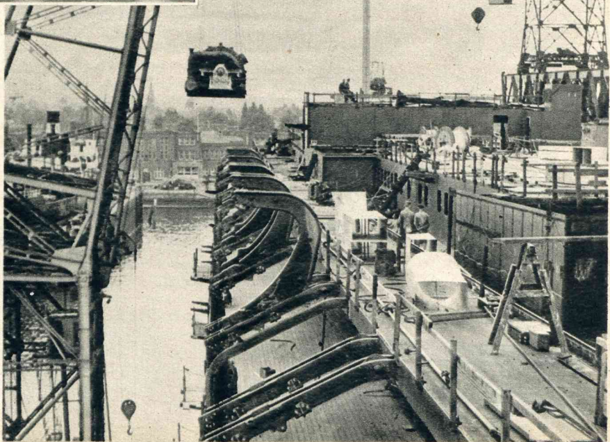
De vorderingen der „Nieuw Amsterdam”. We kiekten op de werf der Rotterdamsche Droogdok Mij. het aan boord hijschen van een der beide lage- en middeldrukturbines der machtige machine-installatie.
