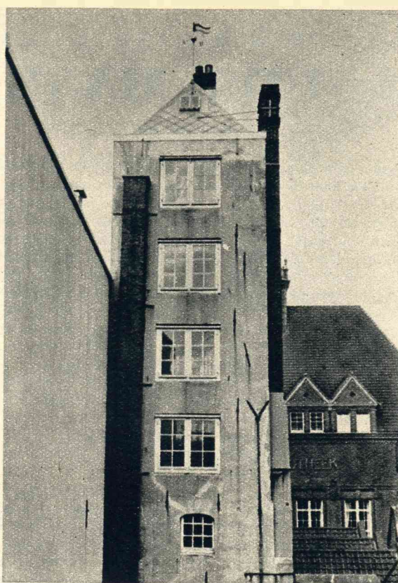
Sedert kort heeft men den ouden z.g. Hageltoren aan de Lombardstraat gerestaureerd. Zooals onze Rotterdamsche lezers wel weten, wordt in dat eigenaardige gebouw een zeer typisch bedrijf uitgeoefend. Daar wordt namelijk de hagel voor jachtpatronen vervaardigd, door gesmolten lood vanuit de hoogste verdieping door een zeef in een lager gelegen waterreservoir te doen vallen. Een buitenaanzicht van de typische fabriek.
