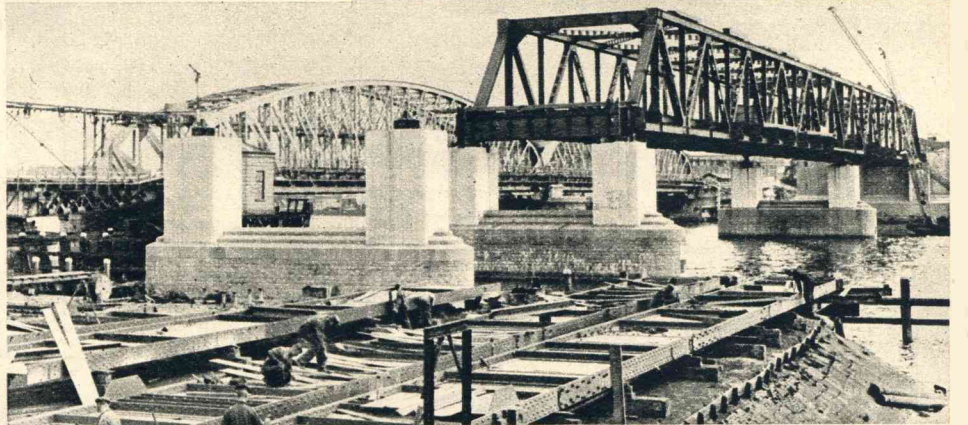
Met den aanbouw der groote verkeersbrug over de Oude Maas tusschen Dordrecht en Zwijndrecht vordert men goed. Het middendeel der brug is reeds gelegd. Men is thans bezig met het samenstellen van het brugdeel aan den Zwijndrechtschen kant.
