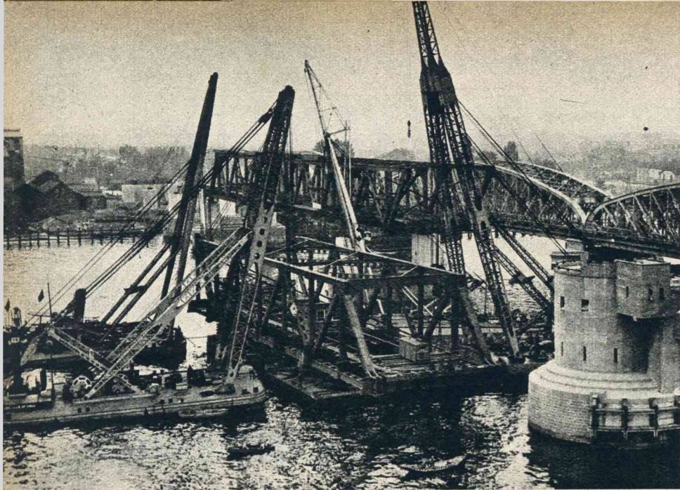
Hoe het groeit! — Een overzicht der vorderende werkzaamheden voor de nieuwe brug over de Oude Maas te Dordrecht. — Moge zij spoedig gereed zijn.
