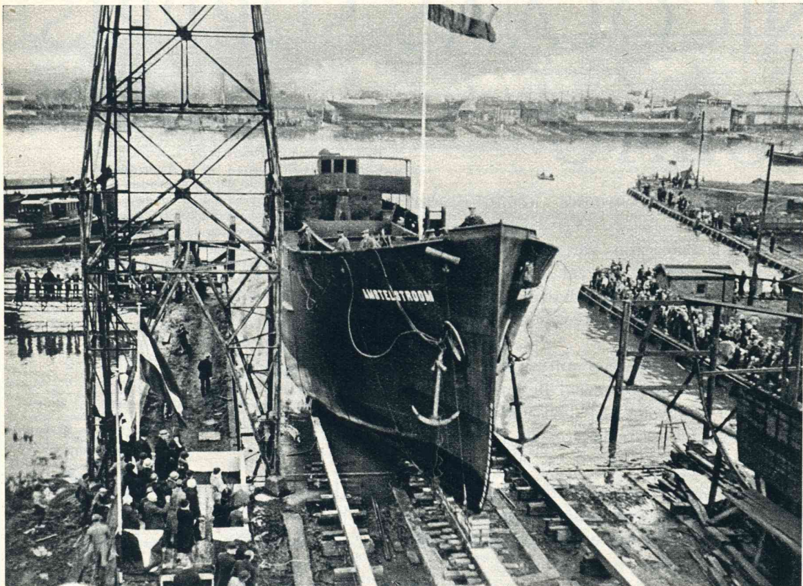
Te Krimpen aan den IJssel werd, van de helling der v. d. Giessen's Scheepswerven, met goed gevolg, te water gelaten het m.s. Amstelstroom, bestemd voor de Holl. Stoomboot Mij., te Amsterdam. — Het schip glijdt in het natte element.
