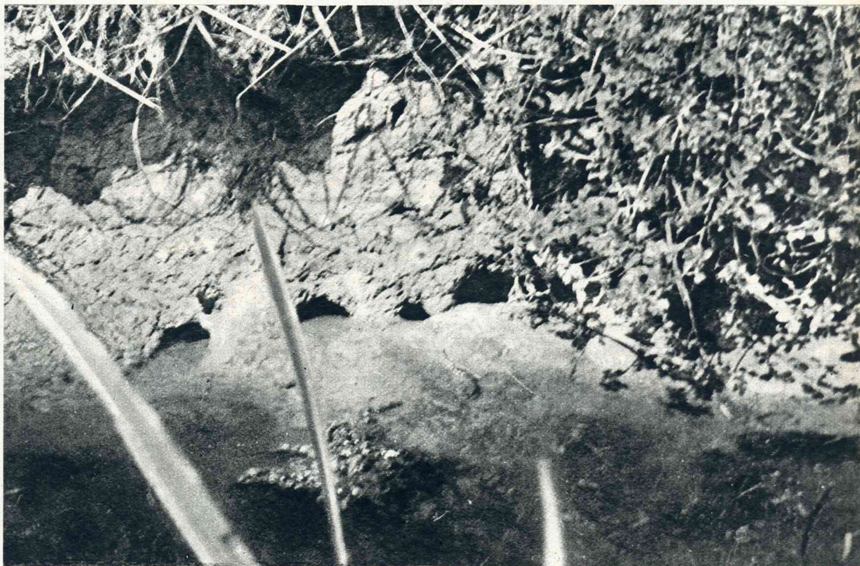
Oeverbeschadiging. Door wolhandkrabben gegraven gaten. Vooral daar waar de oevers uit klei bestaan, kan men deze gaten aantreffen. De lengte is varieerend en bedraagt tot 90 c.M. De doorsnee is ovaal, en de breedte van de gang bedraagt tot 12 c.M. De ingang is trechtervormig verwijd.
