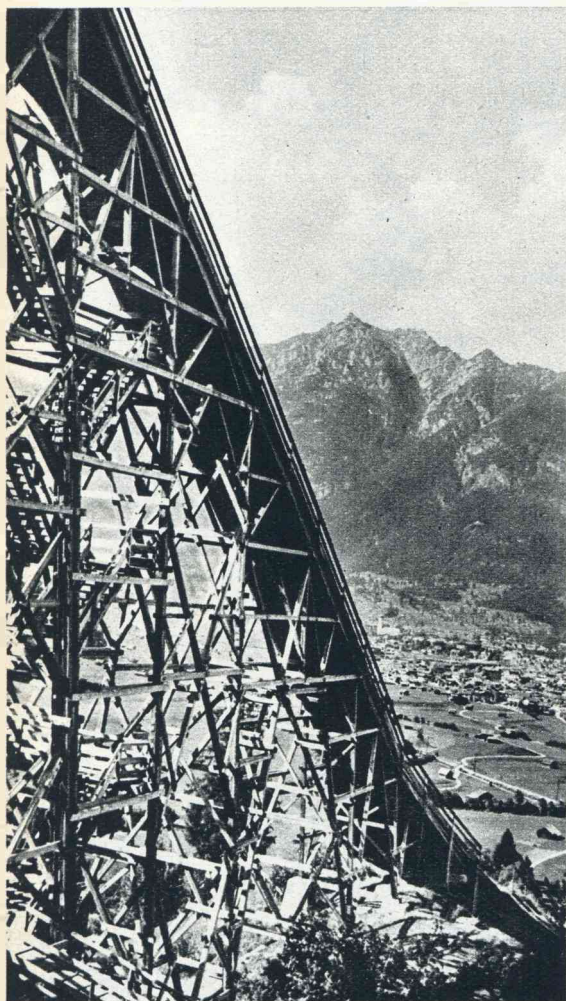
Garmisch is gereed. Kiekje van den 80 M. hoogen springtoren. Hier komen de skispringers in duizelingwekkende snelheid naar beneden om dan een sprong van 80 tot 90 M. in het dal te maken.
