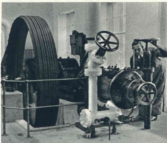
Een der 90 P.K. compressoren, die het ammoniakgas, met behulp waarvan de benodigde koude verwekt wordt, verdichten tot een druk van ongeveer 10 Kilo per vierkanten centimeter. De zuigzijde, waar het koude gas in de machine komt, is geheel met sneeuw, die door de vochtigheid der lucht gevormd wordt, bedekt. De thermometer aan de drukzijde rechts daarentegen toont den monteur, dat hier de temperatuur 83 graden Celsius is, wijl het verdichte gas door de samenpersing sterk verhit werd.
