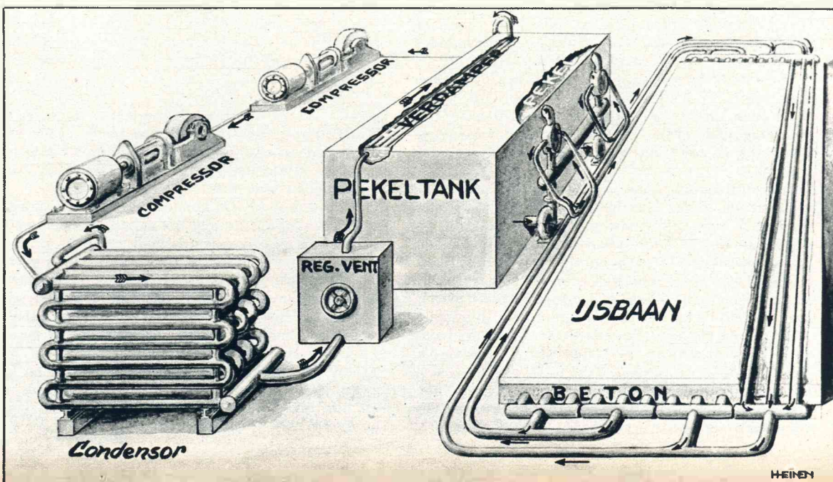
Schema van de installatie met links het eerste en rechts het tweede kringproces. Links boven de compressoren, die het ammoniakgas verdichten, waarna dit via condensor, reguleerstation en verdampers weer bij de compressoren terecht komt. Geheel rechts de betonplaat met daarboren de ijsbaan. De pijltjes geven ook hier aan, hoe de pekels naar het buizenstelsel in de betonplaat gepompt wordt door de pompen, die rechts van de tank afgebeeld zijn, om ten slotte weer naar de tank teruggeleid te worden.
