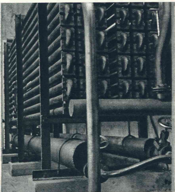
Het regelmatige lijnenspel van den condensor, waar in dubbelwandige buizen het verdichte ammoniakgas door water gekoeld en daardoor vloeibaar wordt.
