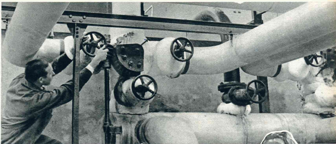
Waar koude gedistribueerd wordt. — Een complex afsluiters, door middel waarvan het mogelijk is de richting, waarin de pekels naar de betonplaat onder de ijsbaan stroomt, om te keeren. Op deze wijze is het mogelijk, steeds dien kant van de baan, die het het meest noodig heeft, de meeste koude toe te voeren.
