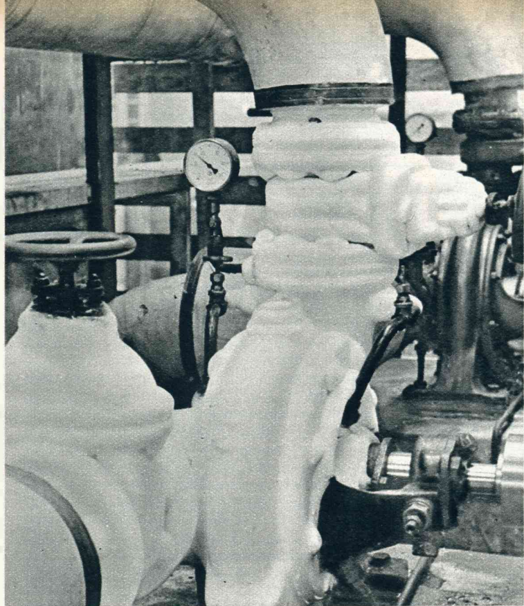
Dit sneeuwtasereel stelt een der pompen voor, die de pekels haar onophoudelijken kringloop doen onderhouden.
