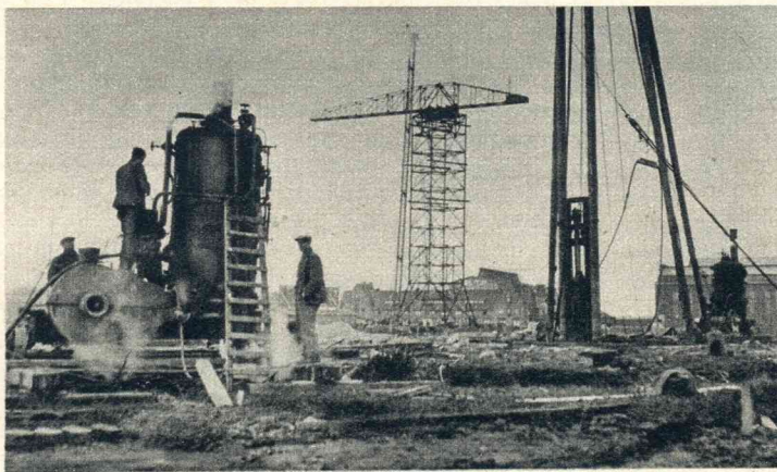
We plaatsen hierbij een aardig kiekje van de voorbereidende werkzaamheden aan het nieuwe Feijenoord-stadion. — Hoe het groeit!
