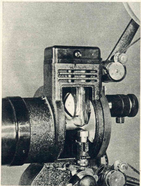
De 16 m.m. smalfilmprojector voor geluidsfilms.
