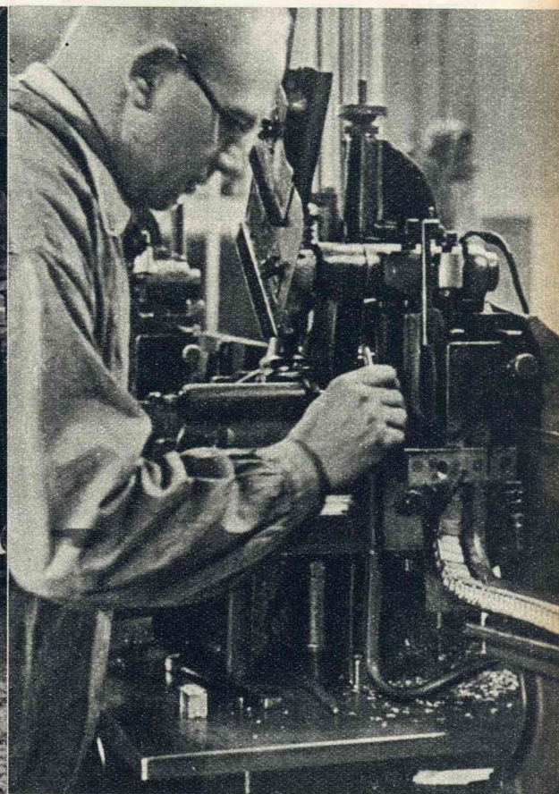
5. De moderne gietmachine stoot in snel tempo een baan gegoten letters uit.
