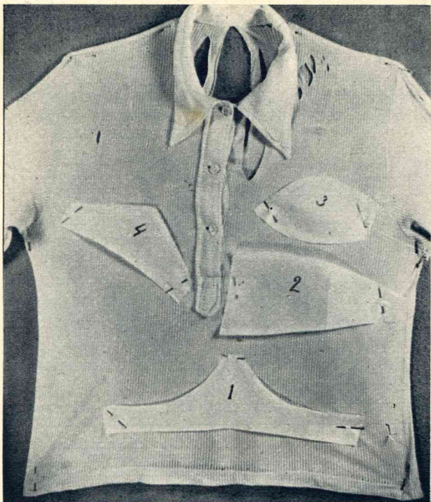
Deel 1, 2 en 3 worden recht geknipt, doch deel 4 schuin.
