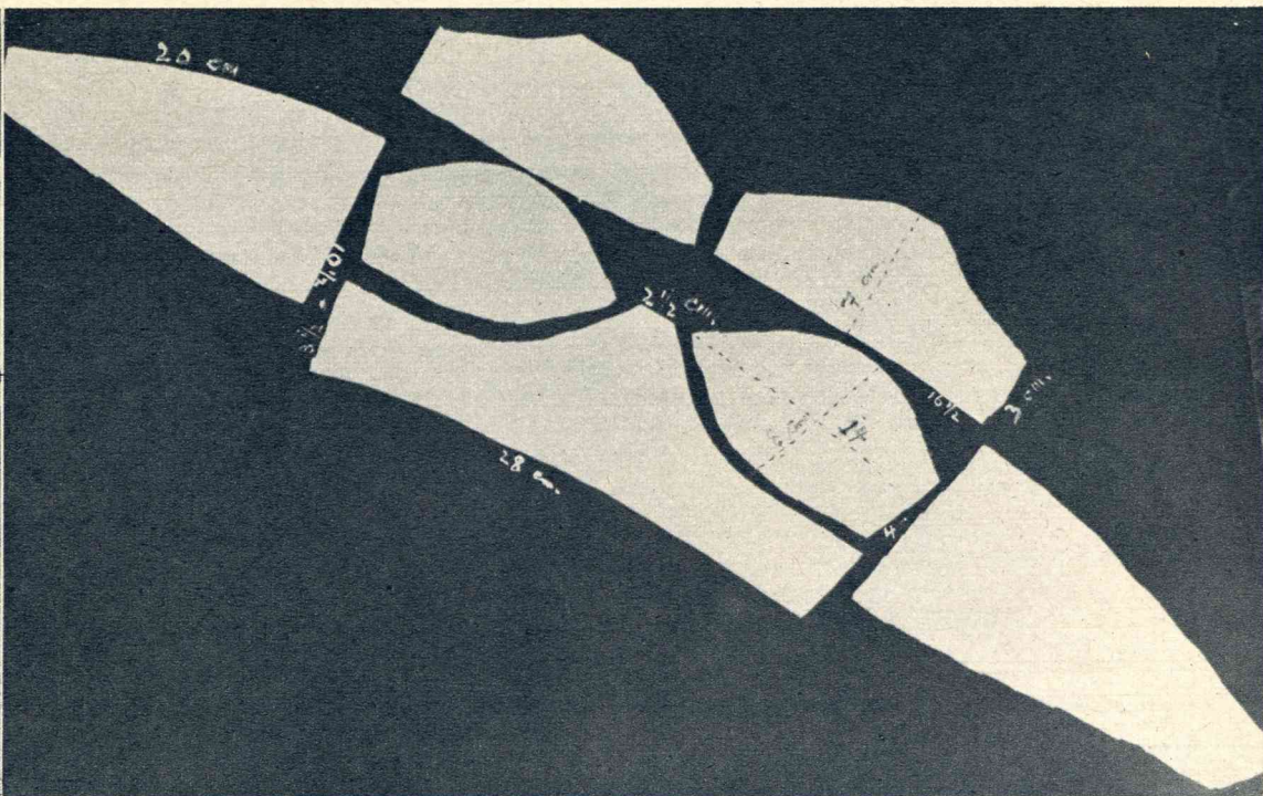
De geknipte delen met hun afmetingen.
