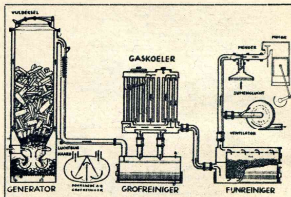
Schema van een generatorinstallatie — in dit geval voor hout — waaruit de lezer een globaal idee van de werking en constructie zal kunnen krijgen. Het gas, in den generatorhaard gevormd door verbranding van het hout met de aangezogen lucht, stroomt — zie de pijltjes — door een grofreiniger, een koeler en een fijnreiniger naar de menginrichting, en vandaar naar den motor. De aanjaagventilator zuigt, bij het starten, gas aan zolang de motor niet draait. Bij de meeste anthracietgeneratoren bestaat de fijnreiniger uit een grooten ketel met filterdoeken.
