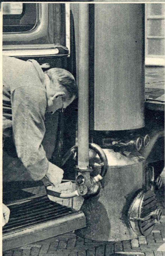
De vuurhaard van een gasgenerator moet 's morgens met een brandende lont worden aangestoken. Een electrische ventilator zuigt de vlam naar binnen.
