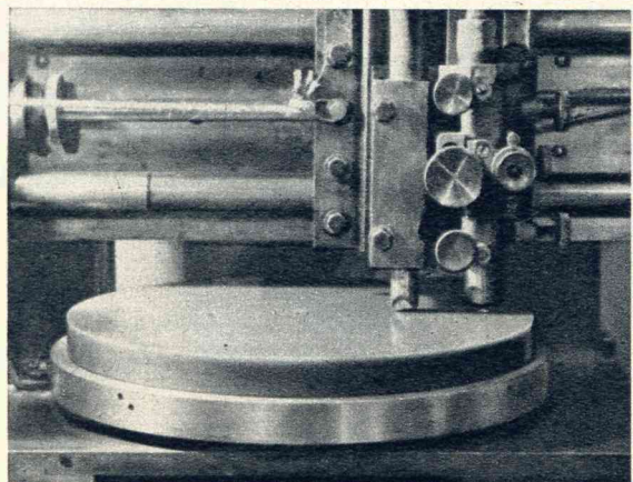
De wasplaat, waarop straks zal worden opgenomen, wordt na het gieten eerst geschaafd en fijn gepolijst.
