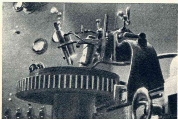
De opname op de wasplaat. De opnamemachine draait, op den achtergrond de versterker. Voorgrond links de microscoop, waardoor de gesneden groeven worden gecontroleerd. Het graveeren van de geluidstrillingen in de wasplaat gebeurt met behulp van een saffier.
