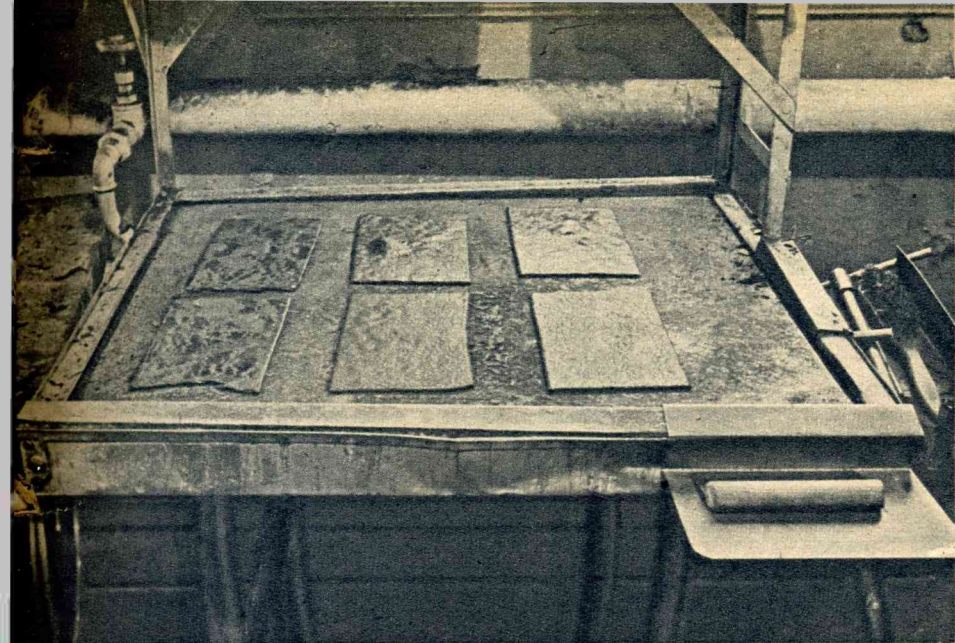
De grondstoffen waaruit de gramfoonplaat bestaat worden gemengd en tot tabletten gevormd. Voor de verdere bewerking worden deze tabletten verwarmd, zoodat ze soepel worden.
