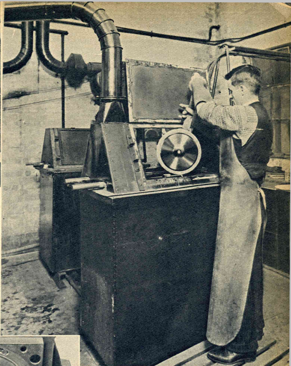
De grondstoffen waaruit de gramfoonplaat bestaat worden gemengd en tot tabletten gevormd. Voor de verdere bewerking worden deze tabletten verwarmd, zoodat ze soepel worden.
