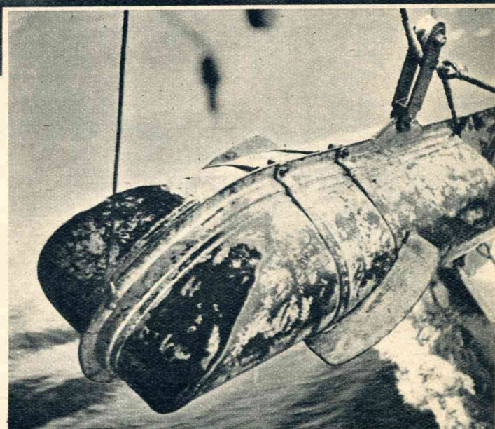
Een close-up van de boei, die achter het schip aan sleept, en waaronder zich de vlieger bevindt; deze laatste zorgt ervoor, dat het zoektuig op een bepaalde diepte „steekt”.
