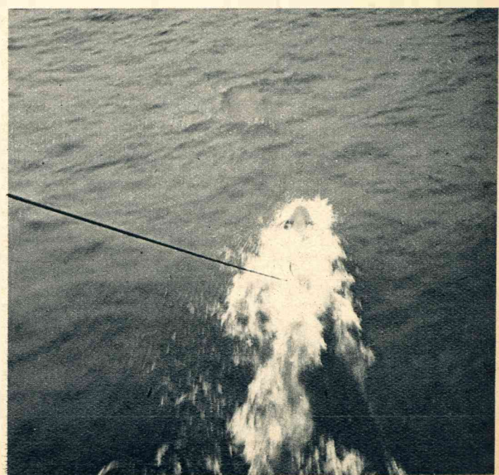
Een close-up van de boei, die achter het schip aan sleept, en waaronder zich de vlieger bevindt; deze laatste zorgt ervoor, dat het zoektuig op een bepaalde diepte „steekt”.
