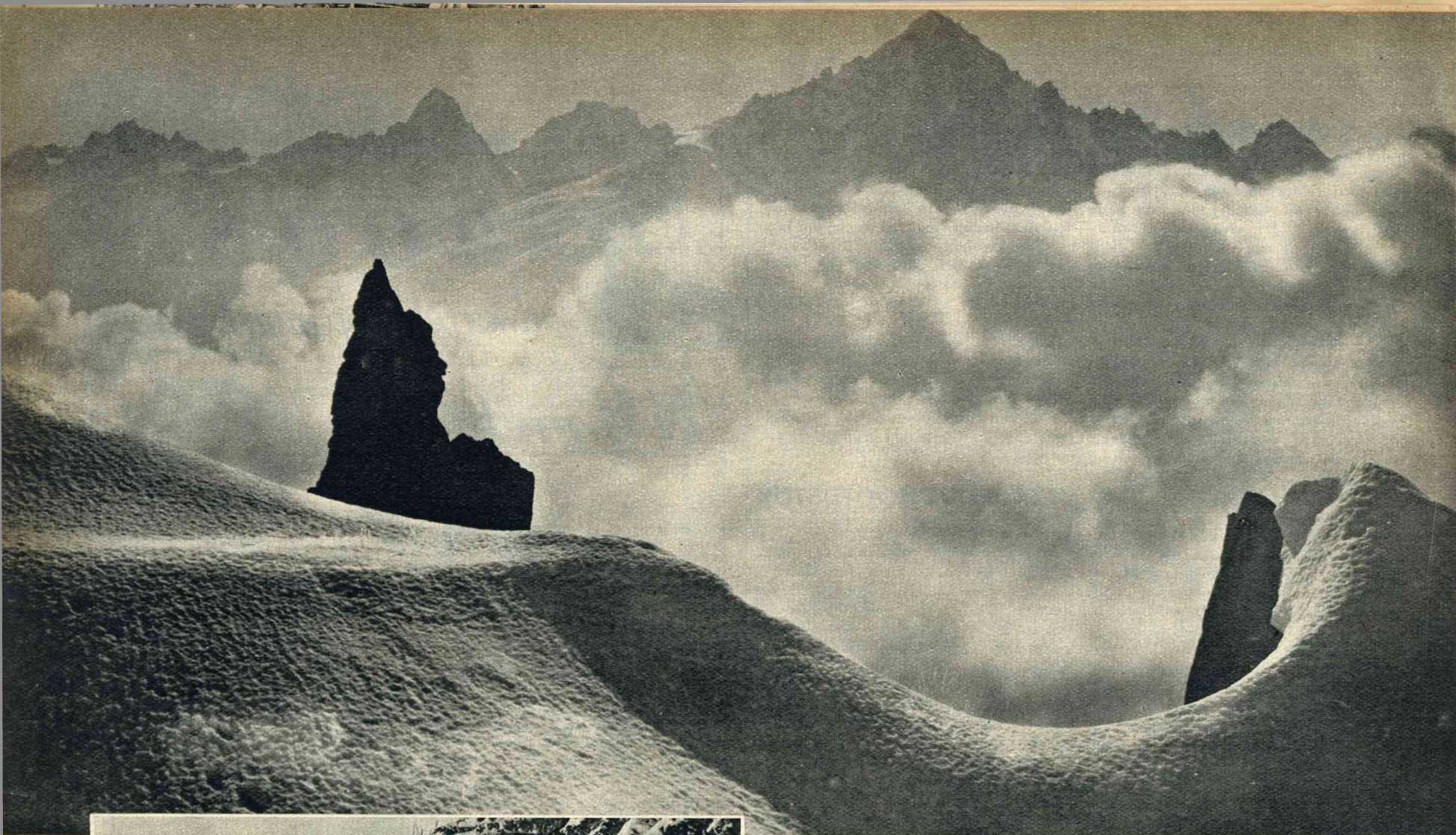
Wolkenspel rond den Aiguille du Dru.
