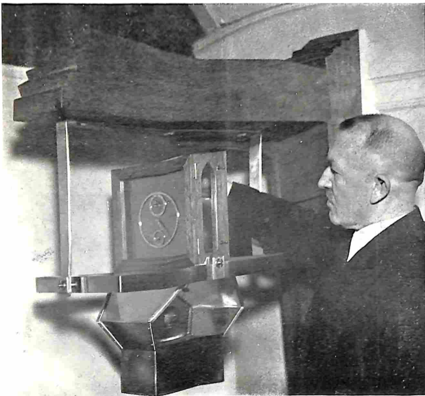
DE RECONSTRUCTIE VAN CHRISTIAAN HUYGENS' TIJDMETER IN HET NEDERLANDSCH HISTORISCH SCHEEPVAART MUSEUM TE AMSTERDAM
