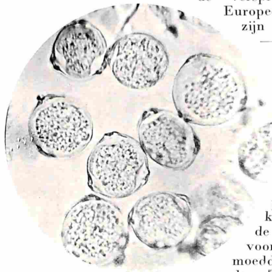
LINKS STUIFMEEL VAN DE ELS, ± 550 × VERGROOT. RECHTS VAN DEN BERK, 625 × VERGROOT
