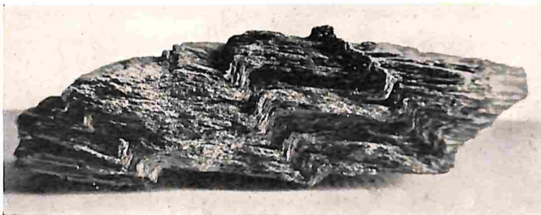
GEPLOOIDE GLIMMERSCHIST (GEVONDEN BIJ MAARN)
