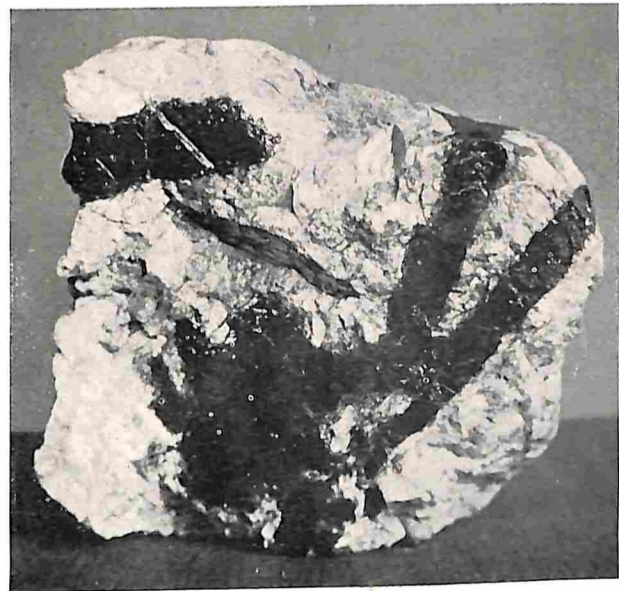
MICA IN GRANIEET (GEV. BIJ AMERSFOORT)
