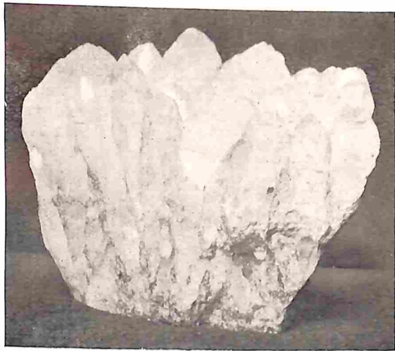
BROK BERGKRISTAL VAN DE VELUWE
