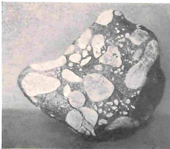
Z.G.N. PUDDINGSTEEN (KIEZEL IN KIEZEL)
