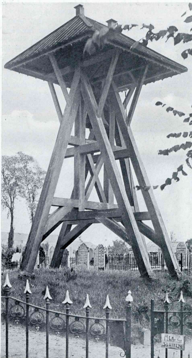
Foto R. H. Herwig KLOKKESTOEL OP HET KERKHOF TE DRACHTEN
