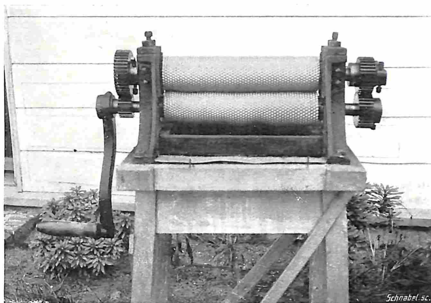
WALSMACHINE VOOR HET VERVAARDIGEN VAN KUNSTRAAT.
