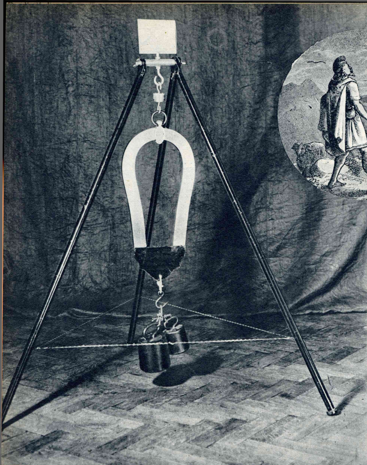
Een oude hoefmagneet (eigen gewicht 10 kg) draagt maximaal 25 kg. Het totaal wordt gemakkelijk gedragen door een magneetje van 100 gram eigen gewicht uit Ticonal 3,8.
